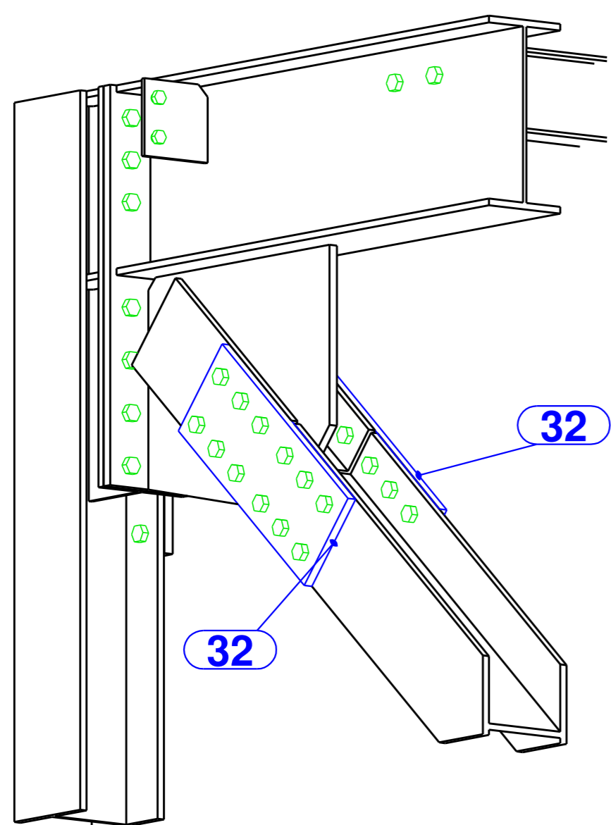
DETALLE UNIÓN-CUBREJUNTAS Marca 32 1:10
